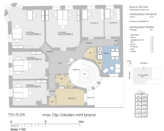
Kv Sjömannen 5 Förslag planlösning, Lokal 31-0401, ca 181 kvm, plan 3tr
